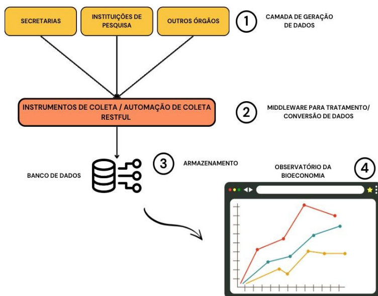
Figura 2. Processo de geração dos dados nos colaboradores, aquisição, tratamento e conversão para o banco de dados estruturado e apresentação dos resultados em um sistema web do Observatório da Bioeconomia.
